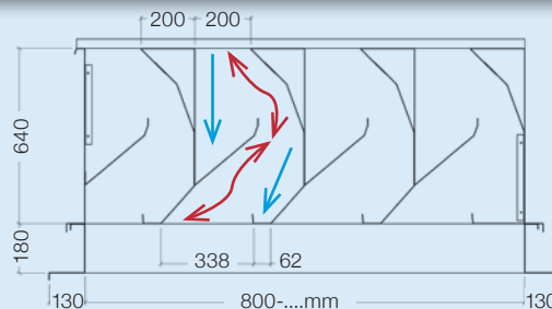
Längsschnitt
