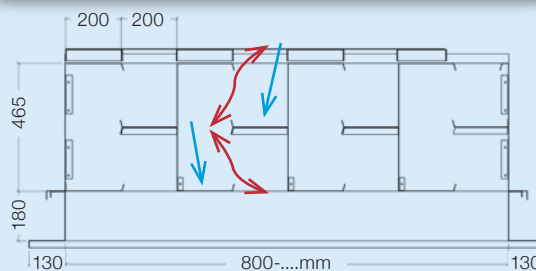
Längsschnitt
